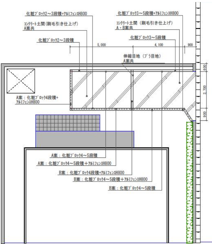
配置図 *現場状況により変更あります。寸法は、概寸になります。
